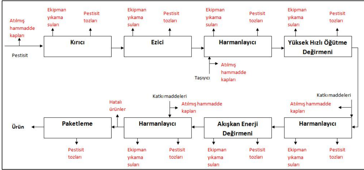
Şekil 57. Kuru böcek ilacı kemirgen ilacı, küf ve mantar ilacı, yabancı otları mücadele ilacı üretimi atık oluşum noktaları
