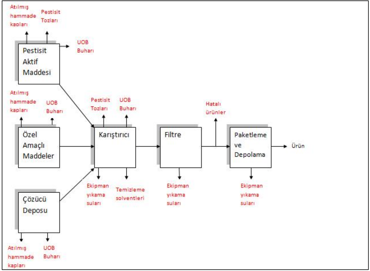
Şekil 56. Sıvı böcek ilacı kemirgen ilacı, küf ve mantar ilacı ve yabancı otları mücadele ilacı üretimi atık oluşum noktaları
