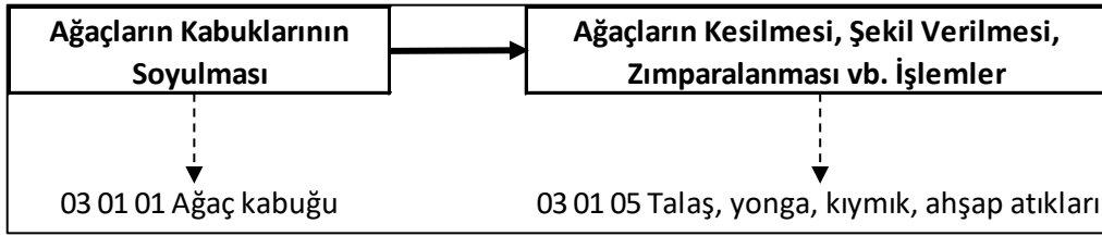
Şekil 35. Ham ağaç ürünleri üretimi atık oluşum noktaları
