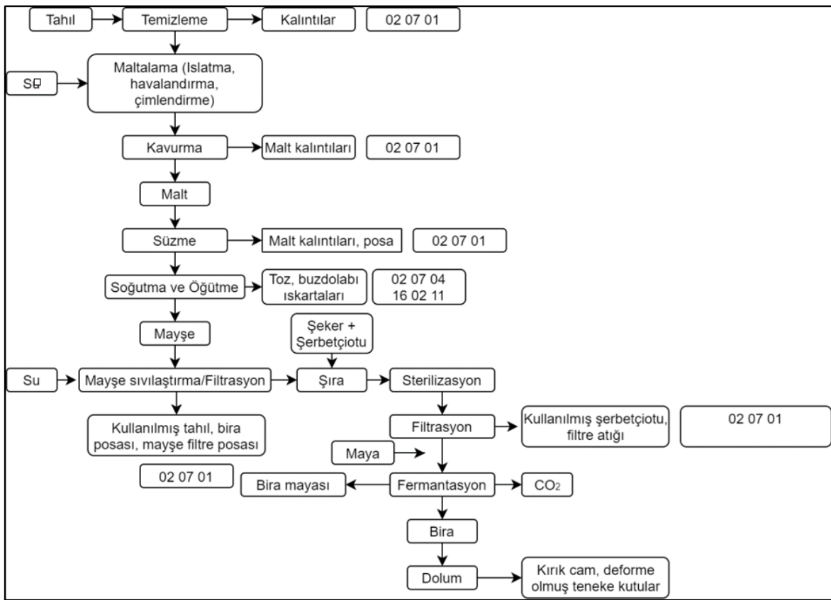
Şekil 6. Bira üretimi akım şeması ve kaynaklanan proses atıkları 24
