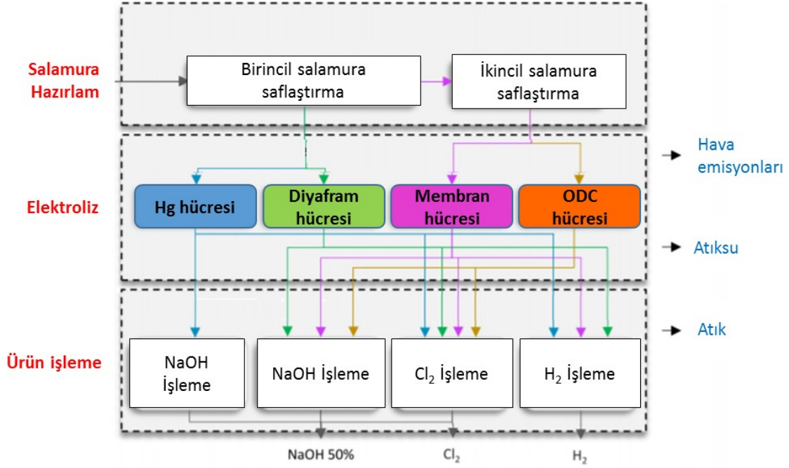
Şekil 49. Klor-alkali prosesleri 61
