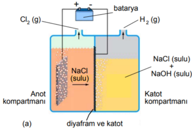
Şekil 52. Diyafram hücresi 64
