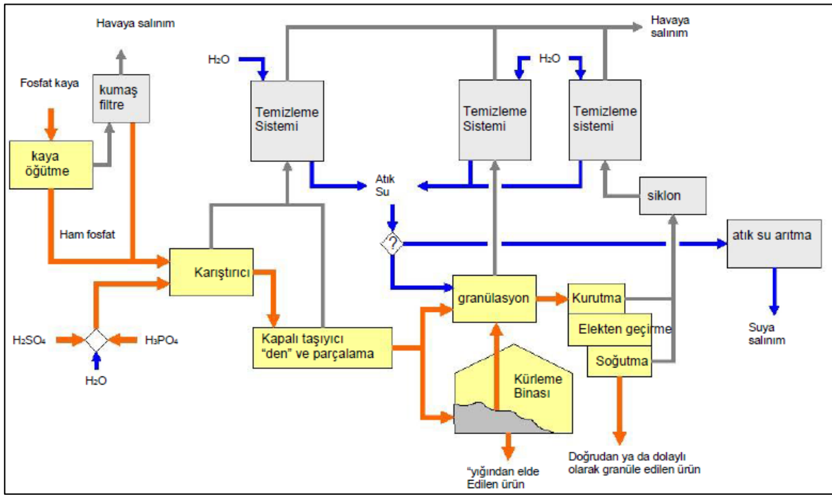
Şekil 55. Süper fosfat üretimi hakkında genel prosesler (atık gaz artıma sistemi dahil)
