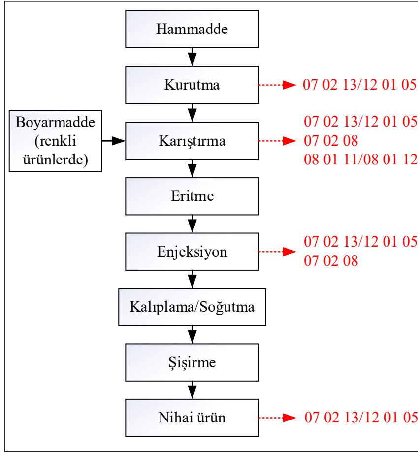
Şekil 70. Plastik şişe üretim aşamaları ve atık oluşum noktaları
