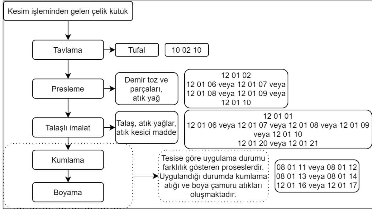
Şekil 79. Çelikten yapılmış tüp, boru, içi boş profiller ve ilgili bağlantı parçalarının üretim proses akım şeması ve oluşan atıklar
