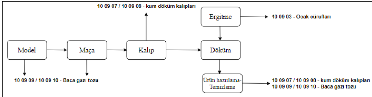
Şekil 83. Demir döküm tesislerinde atık oluşum noktaları
