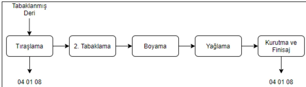
Şekil 34. Tabaklanmış deri işleme sektörü atık oluşum noktaları
