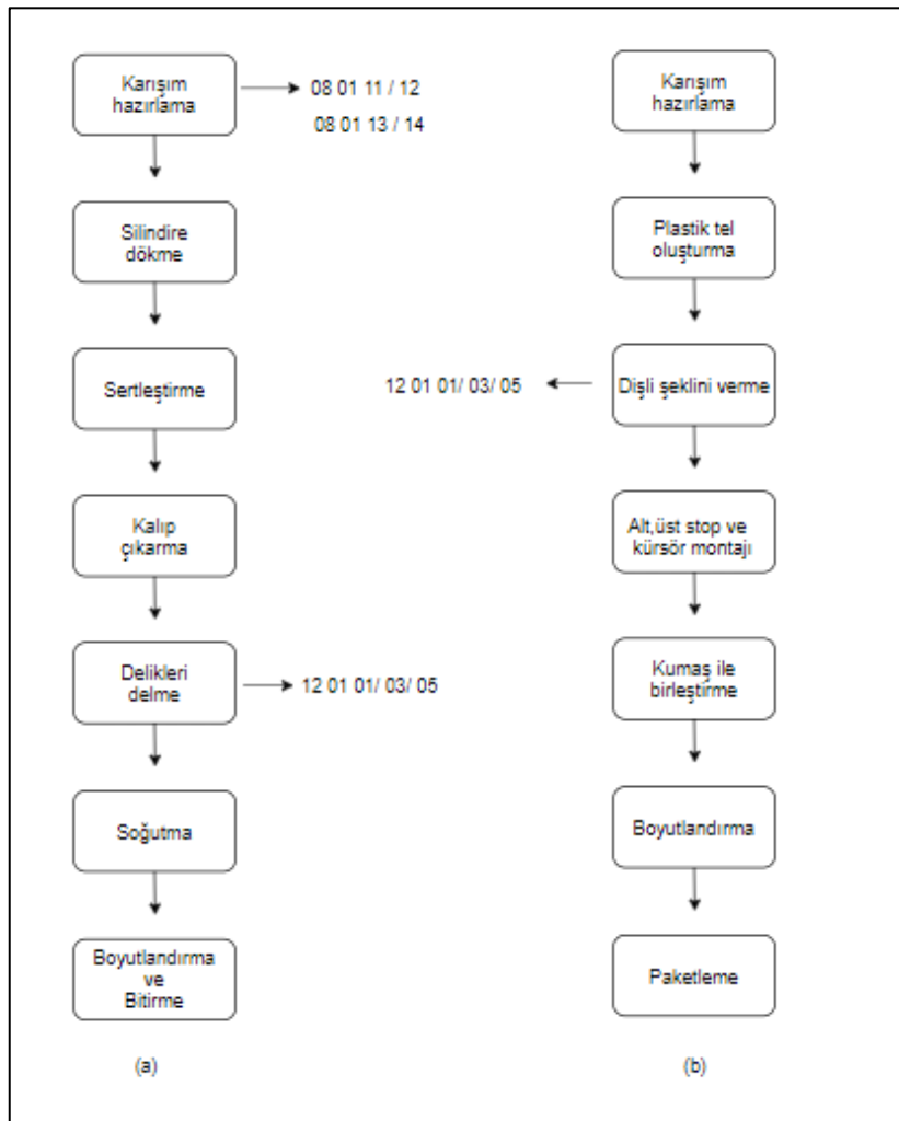
Şekil 101. Kot vb. baskı düğmeleri, çitçitlar, düğmeler, fermuarlar vb. imalatı üretim süreci
