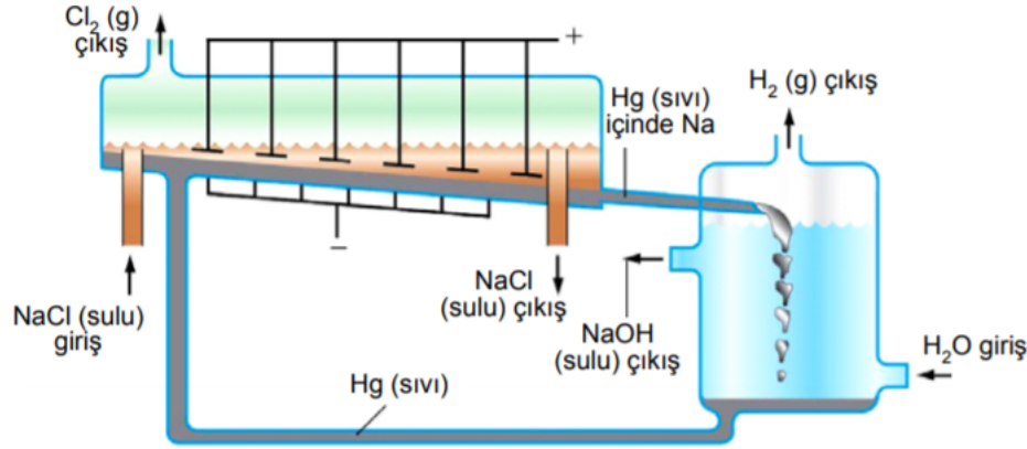
Şekil 51. Cıva hücresi 63
